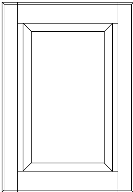
Largeur et hauteur minimum (solide) = 8 1/2" Largeur et hauteur minimum (contreplaqué) = 7 1/2"
