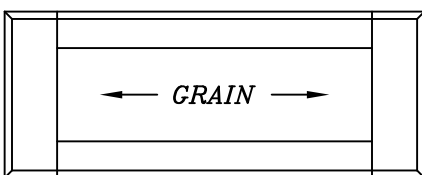
Hauteur minimum disponible = 5 7/8" Largeur minimum disponible = 7 1/4" (Avec panneau visible de 1/8")
