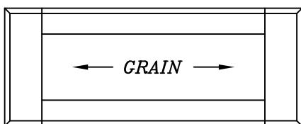
Hauteur minimum disponible = 5 7/8" Largeur minimum disponible = 8 3/4" (Avec panneau visible de 1/8")
