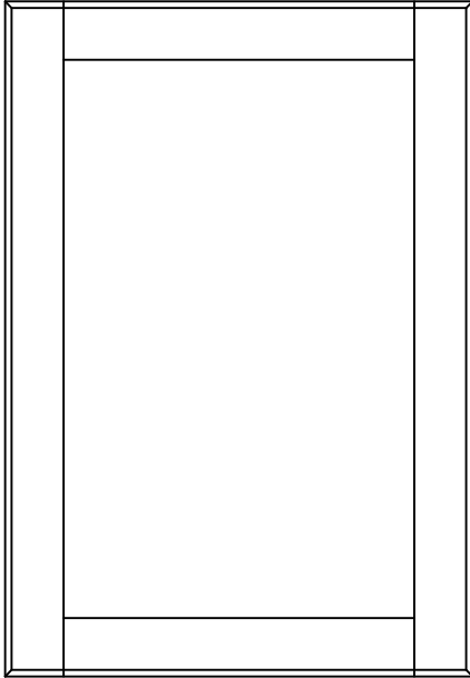
Largeur et hauteur minimum (solide) = 7" Largeur et hauteur minimum (contreplaqué) = 5 5/8"
