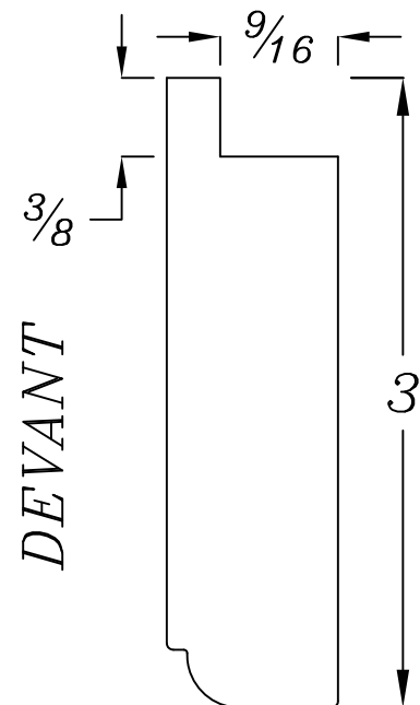
profil extérieur représenté = E-04
