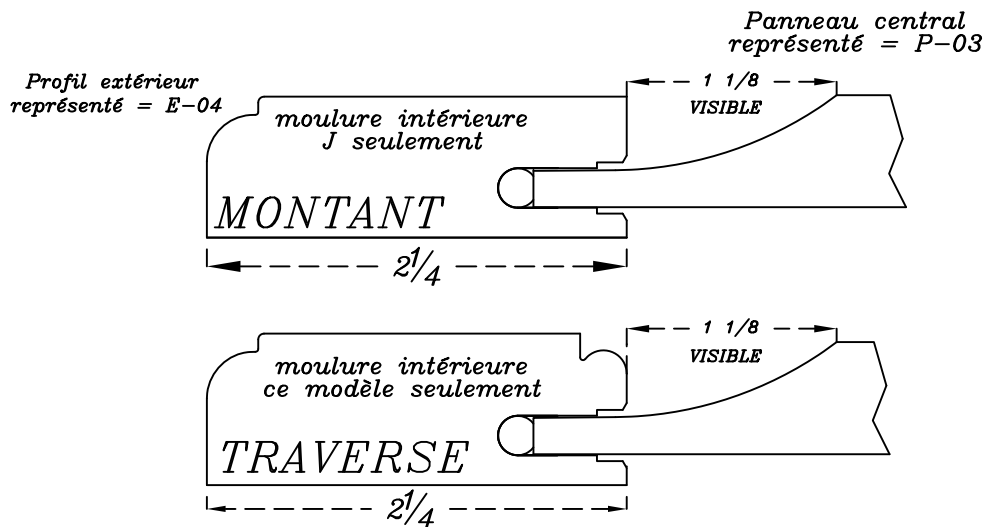
Largeur et hauteur minimum (solide) = 7" Largeur et hauteur minimum (contreplaqué) = 6"
