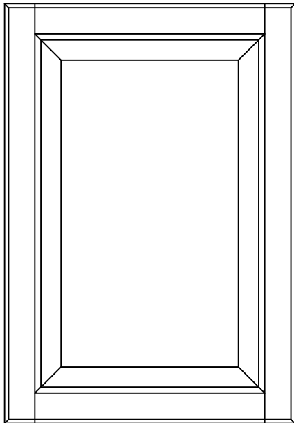
Largeur et hauteur minimum (solide) = 6 1/2" Largeur et hauteur minimum (contreplaqué) = 5 1/8"
