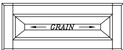
Hauteur minimum disponible = 6 3/4" Largeur minimum disponible = 6 3/4" (Avec panneau visible de 1/8")
