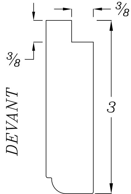
profil extérieur représenté = E-04
