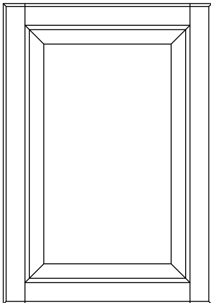
Largeur et hauteur minimum (solide) = 8" Largeur et hauteur minimum (contreplaqué) = 7"
